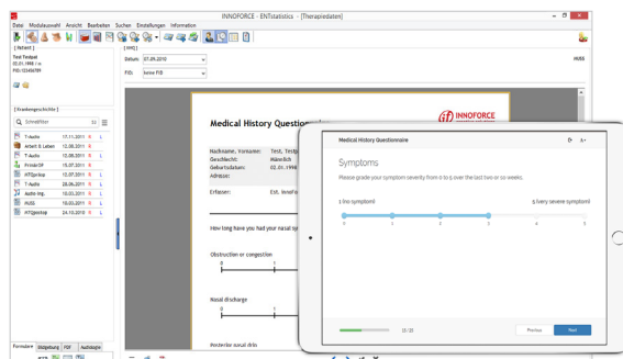
Fragebogen-Funktionalität
